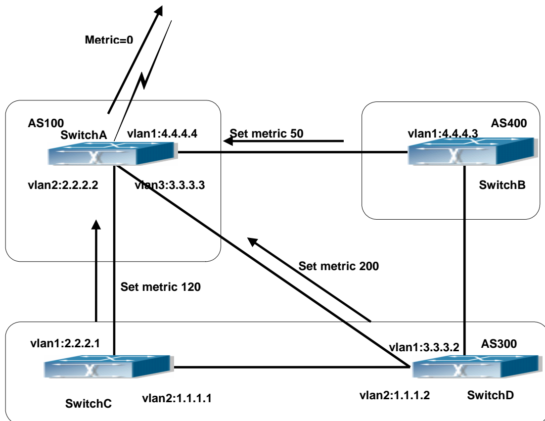
Fig 14-13 MED Configuring Topological Map
