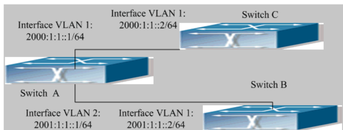
Fig 14-5 RIPng Example
