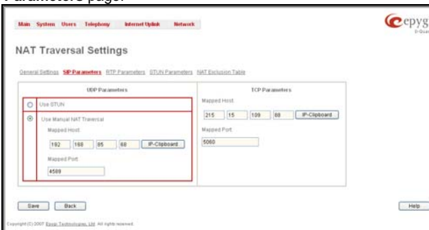
Fig. I- 33: NAT Traversal Settings - SIP Parameters
